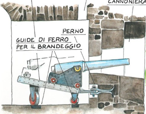
ARTIGLIERIA IN CASAMATTA DEL FORTE DI FENESTRELLE (1728-1837)
