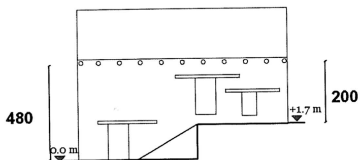
PROSPETTO EST
