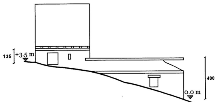
PROSPETTO NORD
