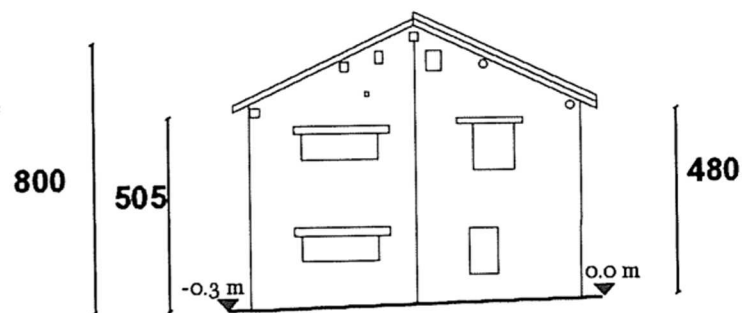
PROSPETTO SUD
