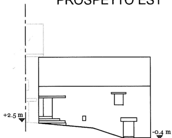
PROSPETTO EST
