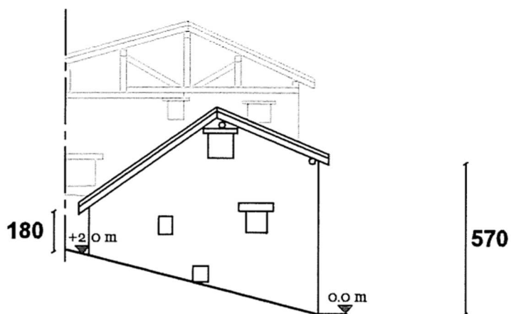
PROSPETTO SUD-OVEST
