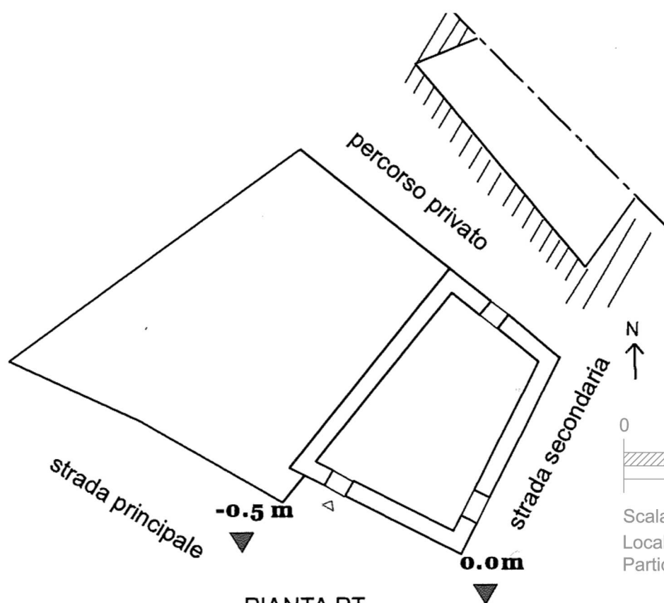
PIANTA PT
