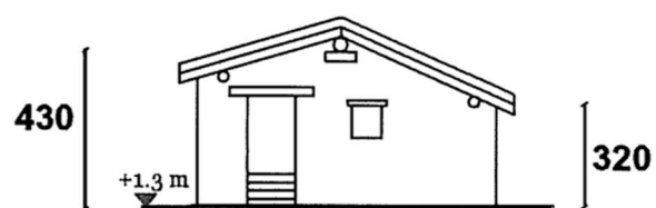
PROSPETTO NORD
