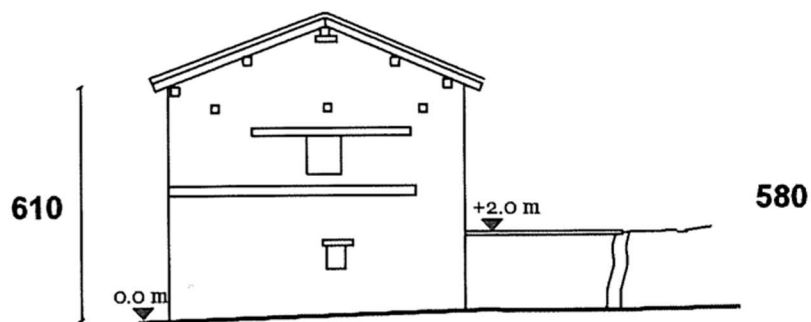
PROSPETTO SUD
