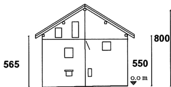
PROSPETTO SUD
