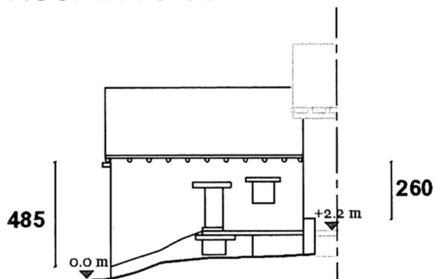
PROSPETTO EST
