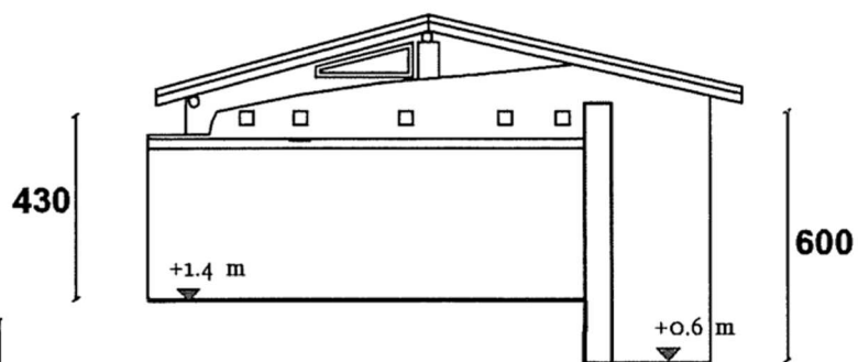
PROSPETTO OVEST
