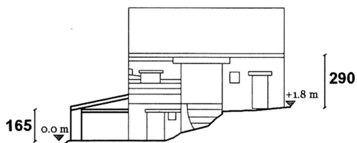
PROSPETTO SUD-EST
