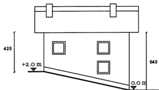
PROSPETTO NORD-OVEST
