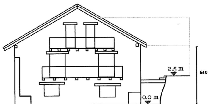
PROSPETTO OVEST
