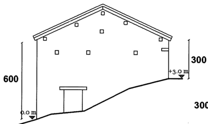
PROSPETTO SUD
