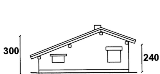
PROSPETTO EST
