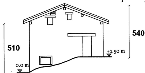
PROSPETTO OVEST
