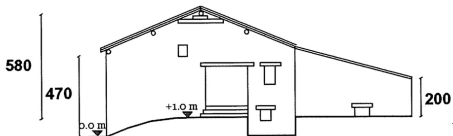
PROSPETTO SUD
