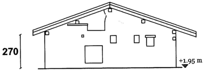
PROSPETTO EST
