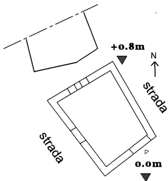
PIANTA PT
