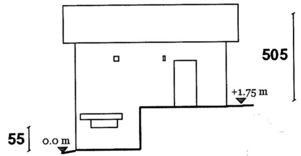
PROSPETTO SUD
