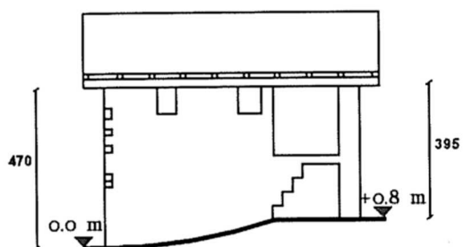
FACCIATA EST
