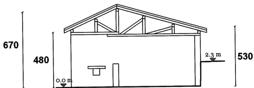
PROSPETTO NORD
