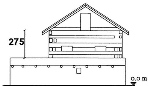
PROSPETTO SUD/OVEST
