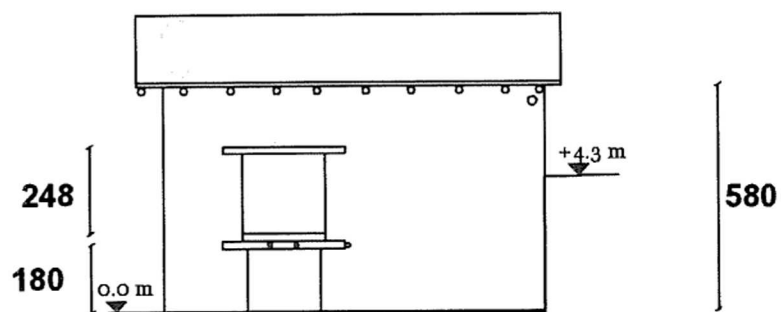
PROSPETTO EST
