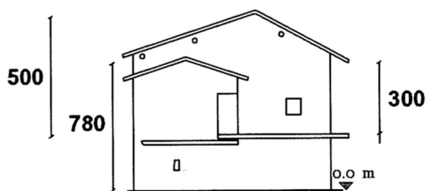
PROSPETTO OVEST
