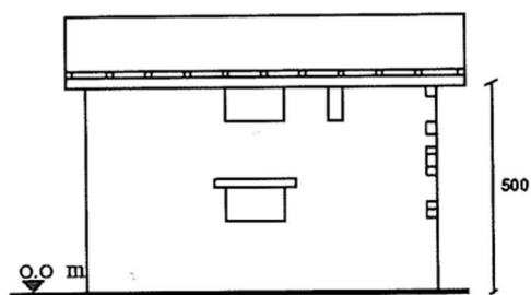
FACCIATA OVEST
