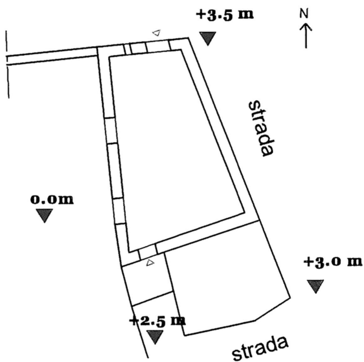
PIANTA 1P
