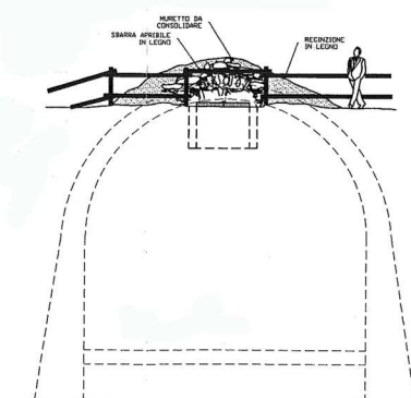
Prospetto Nord
