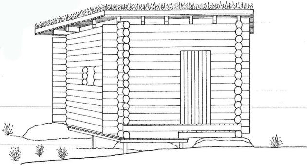
Prospetto Est
