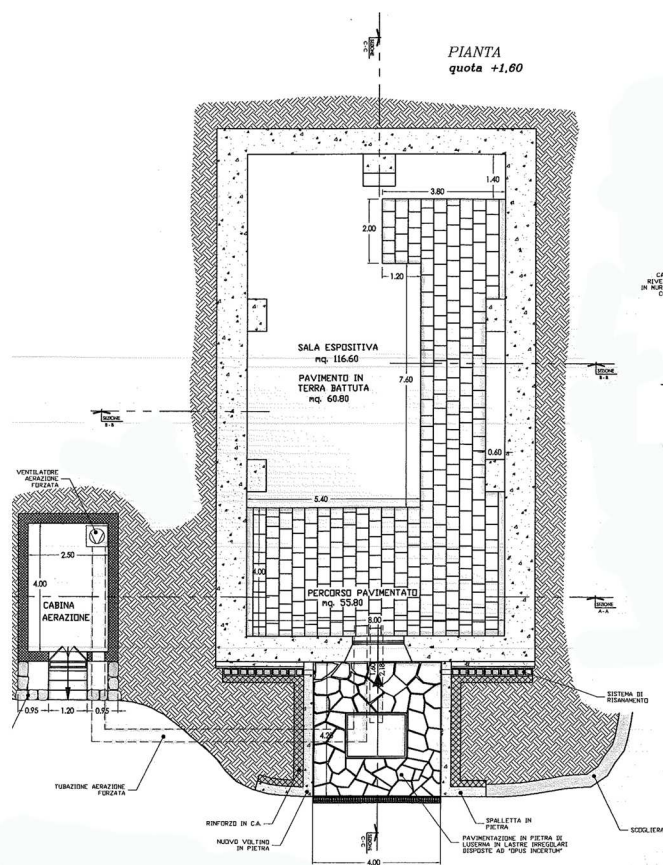
Pianta della Ghiacciaia
