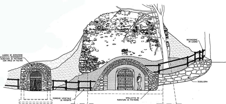
Prospetto Sud
