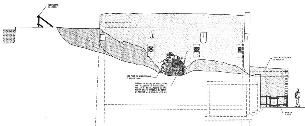
Prospetto Est
