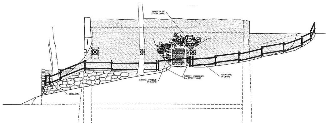
Prospetto Ovest
