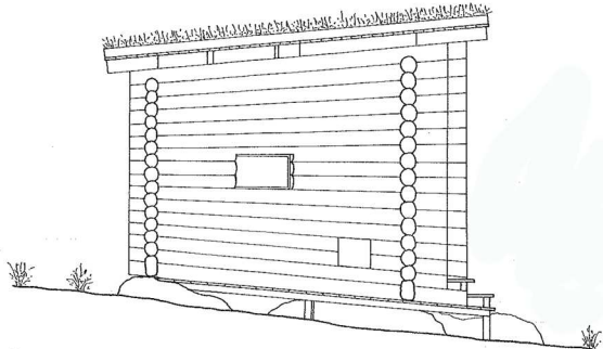
Prospetto Nord
