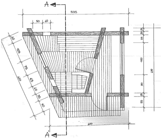
Pianta della Sauna
